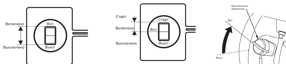
Рис. 15. Выключатель зажигания
